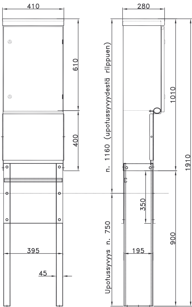
Asennus maahan
