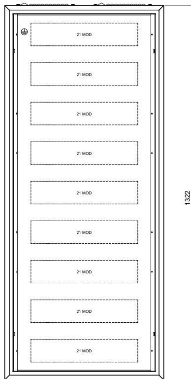
VARMA RX-189C 33 001 52
