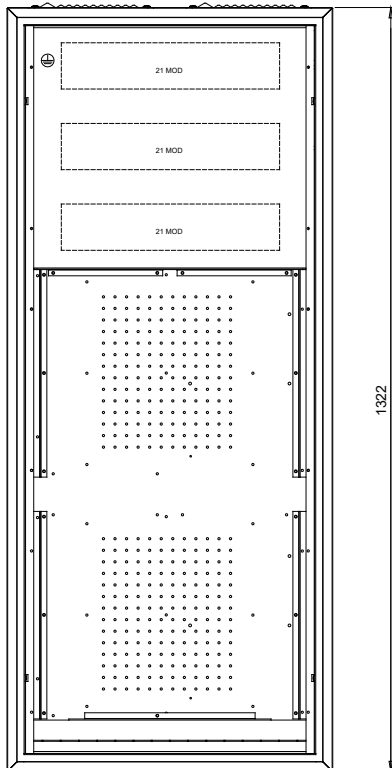
VARMA IT-3C 33 001 42
