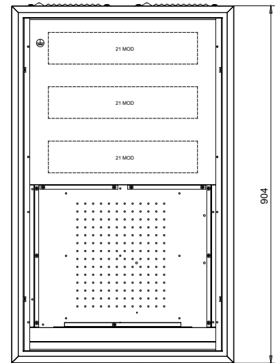
VARMA IT-2B 33 001 41
