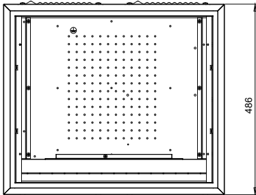
VARMA IT-1A 33 001 40
